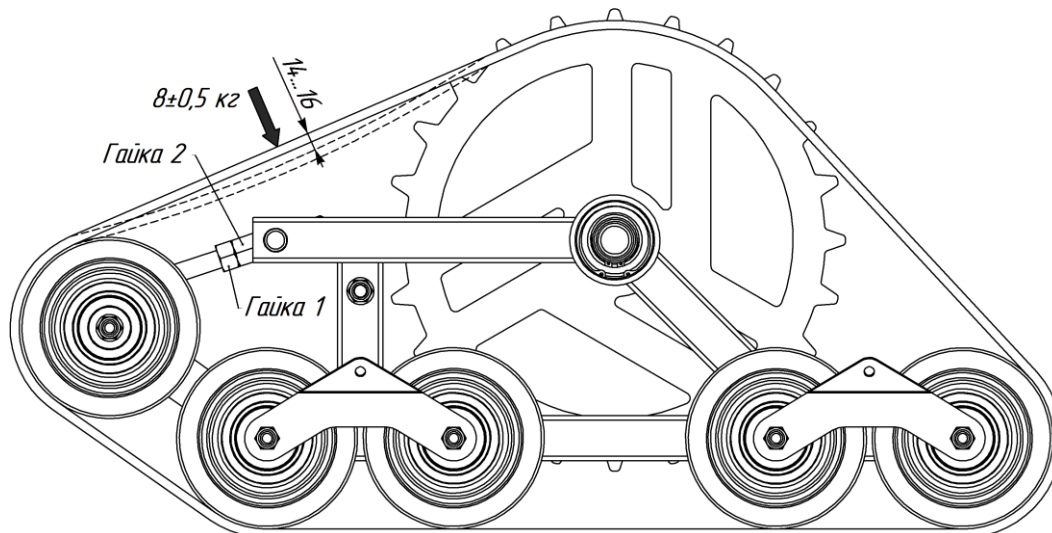
Рис.3. Проверка натяжения гусеницы.
